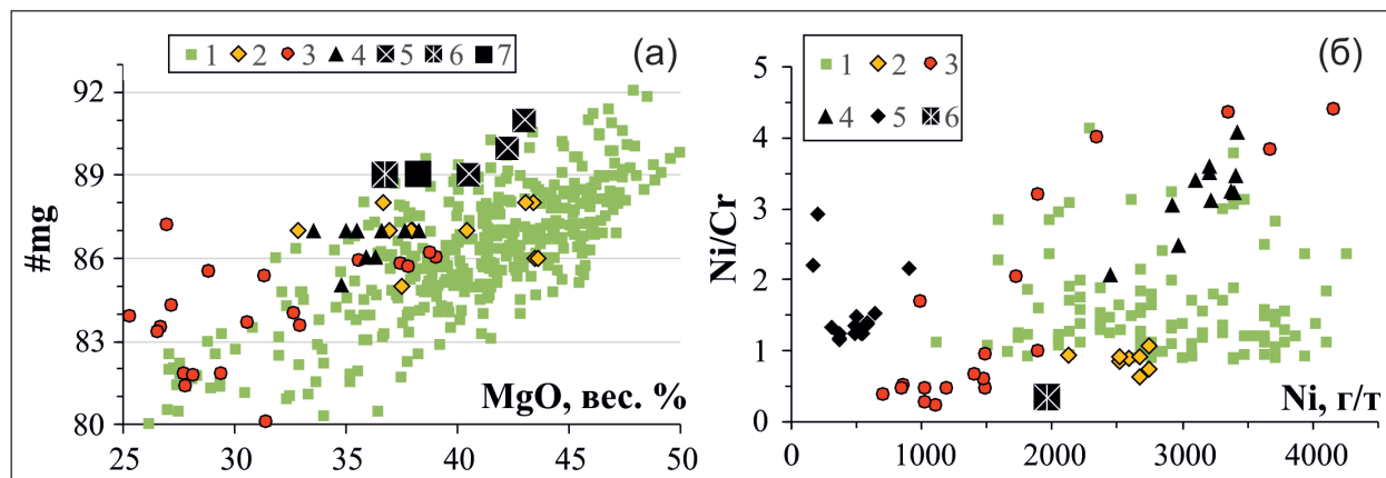
Рис. 2. (а) Соотношение #mg и MgO в ультрамафитах ПГК: 1 – Голованевского домена, 2 – Немировской интрузии (Цымбал и др., 1996), 3 – включений в эндебитах (Лобач-Жученко и др., 2018), 4 – структуры Вредефорт (Hart et al., 1990), 5 – средний состав ксенолитов перидотитов верхней мантии Байкало-Монгольской области (Никитина и др., 2010), 6 – верхняя мантия (Palme, O'Neil, 2014), 7 – деплетированная мантия (Salters, Stracke, 2004). (б) Содержание Ni и Ni/Cr отношение в ультрамафитах ПГК. Знаки 1-4 и 6 – те же, что на рис. (а), 5 – импактные расплавы структуры Мороквенг (Andreoli et al., 1999).
